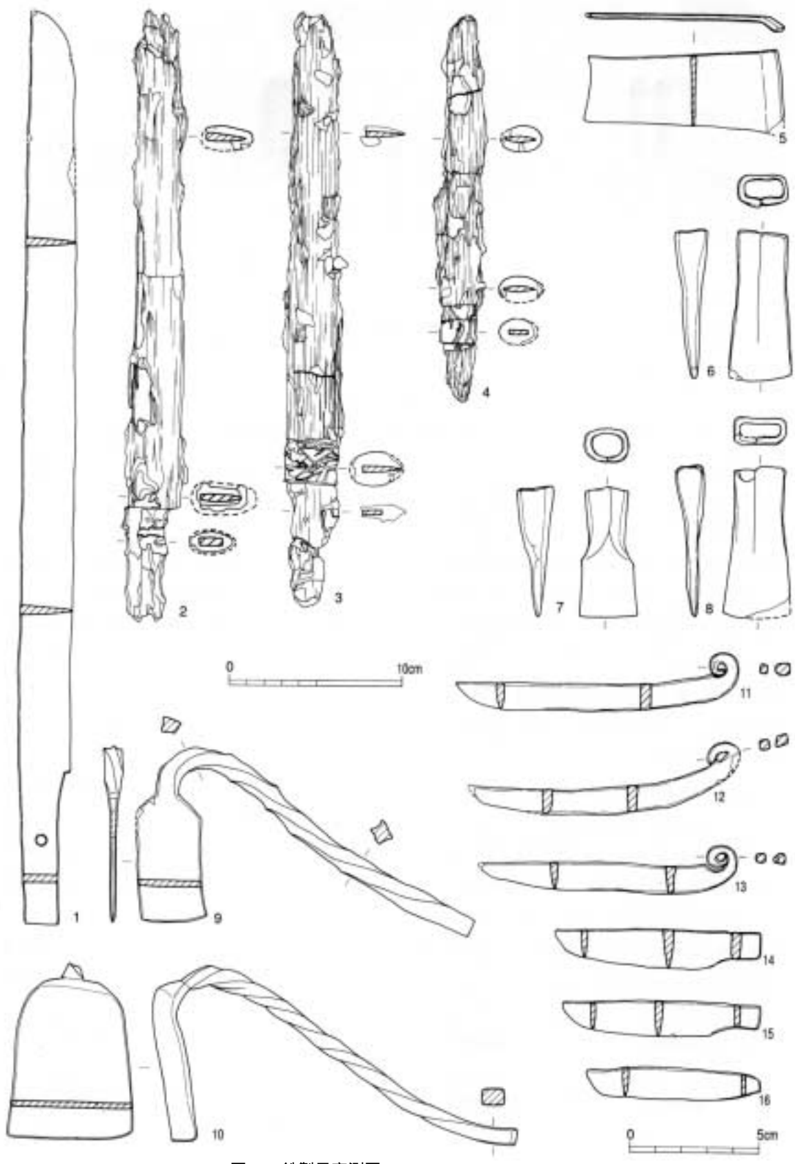
图14 鉄製品実測図 (1~4S:1/3, 5~16S:1/2) 1~3刀, 4剣, 5鎌, 6~8斧, 9柄付縦斧, 10柄付横斧, 11~13蕨手刀子, 14~16刀子
