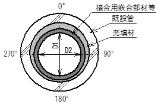
図 参 6-7-1 仕上がり内径を測定する位置
