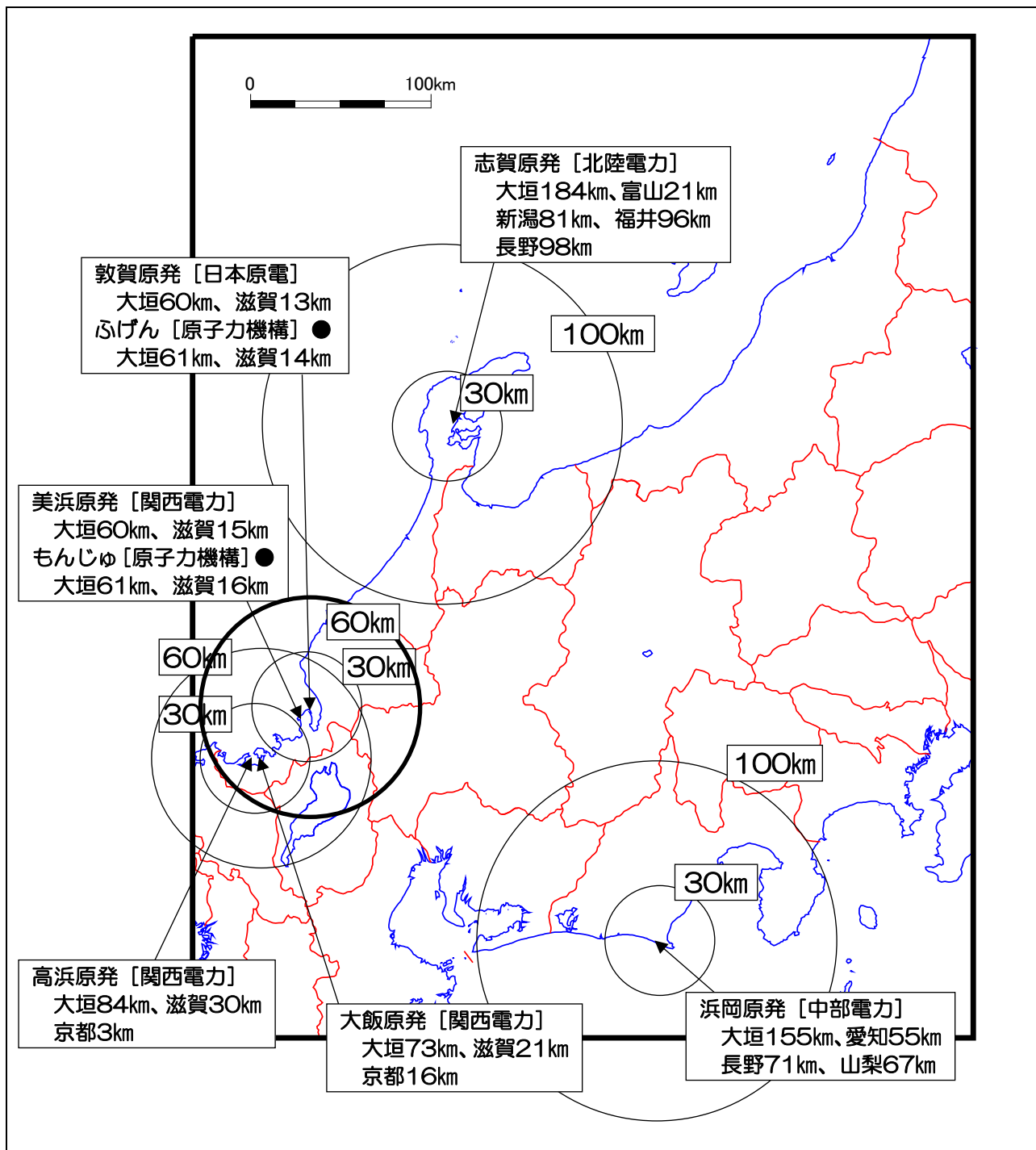
〔大垣市周辺の原子力事業所位置図〕
