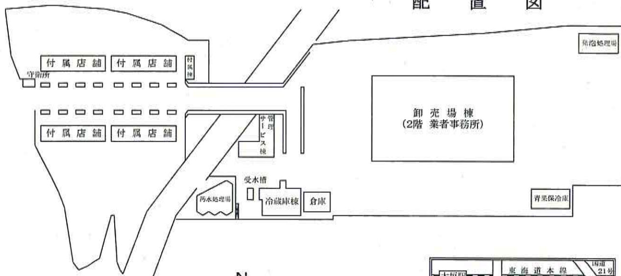
配 置 図
