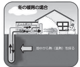
地下水利用地中熱ヒートポンプのしくみ
